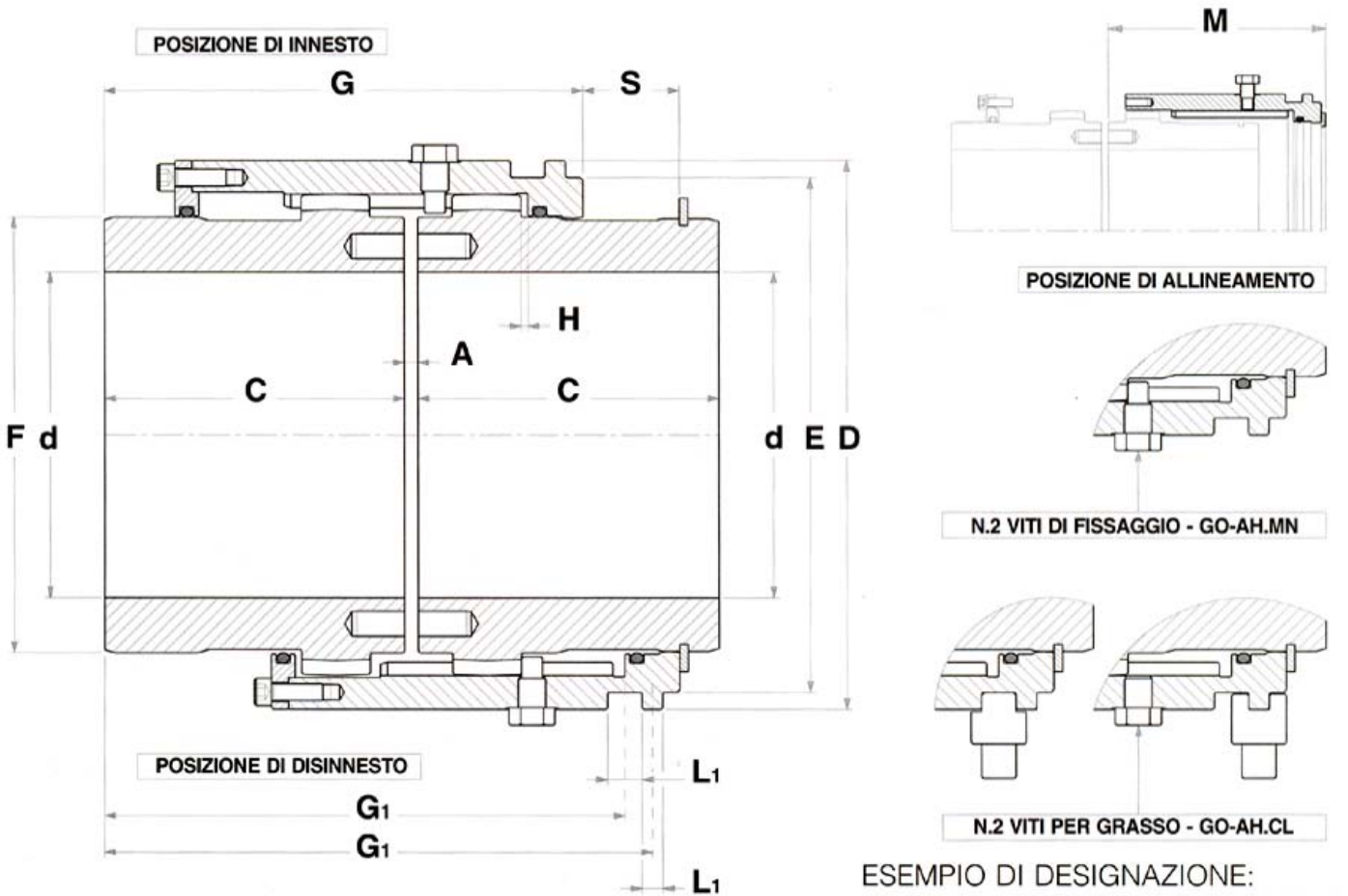
Fig. 28 - Giunto GO-AH.MN
