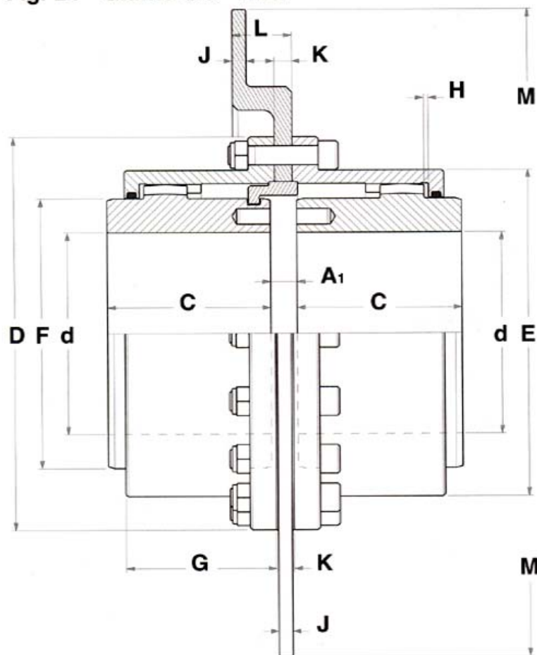
Fig. 25 - Giunto GO-A.DF
