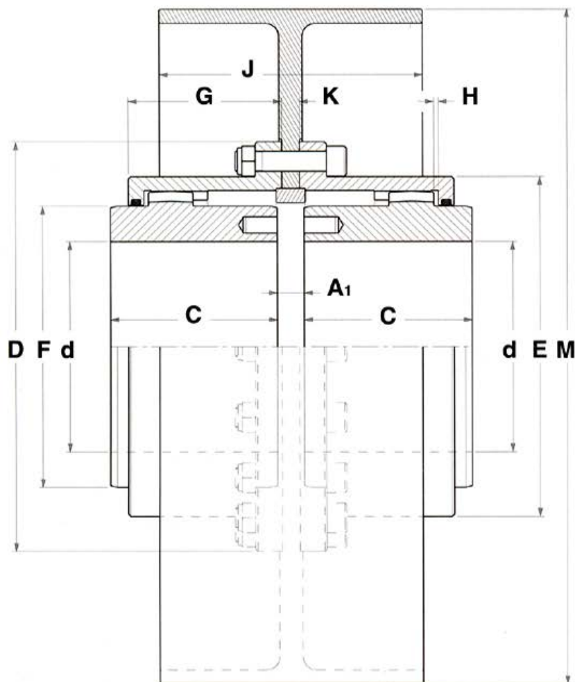
Fig. 23 - Giunto GO-A.FF
